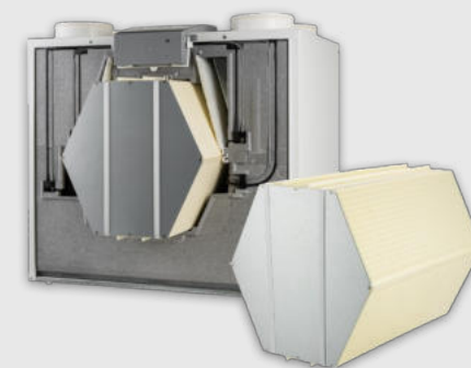
ENTHALPIEWISSELAAR
